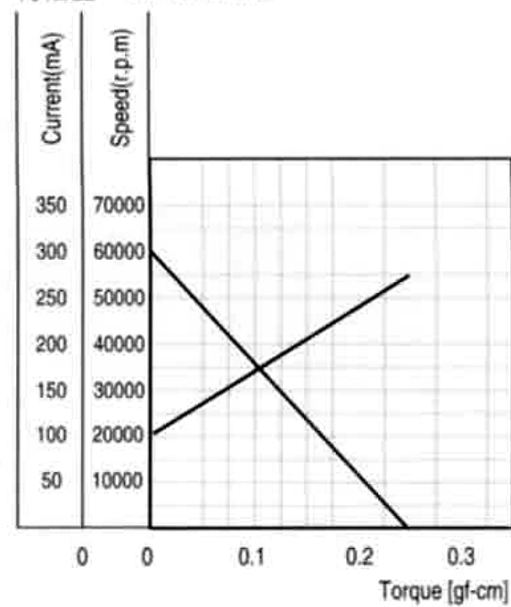
特性图 Characteristics
