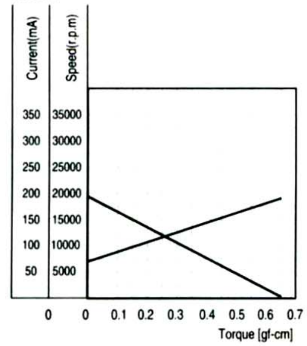
特性图 Characteristics
