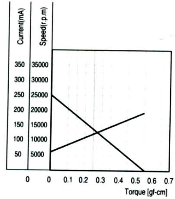
特性图 Characteristics
