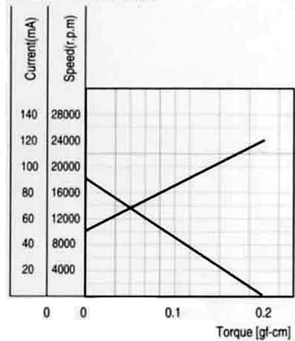
特性图 Characteristics
