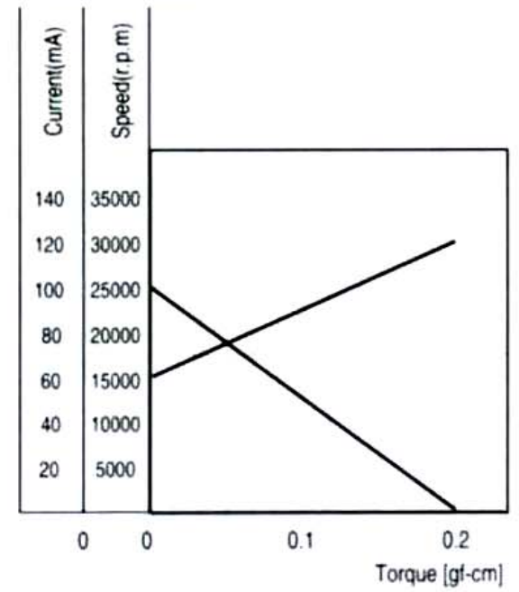
特性图 Characteristics
