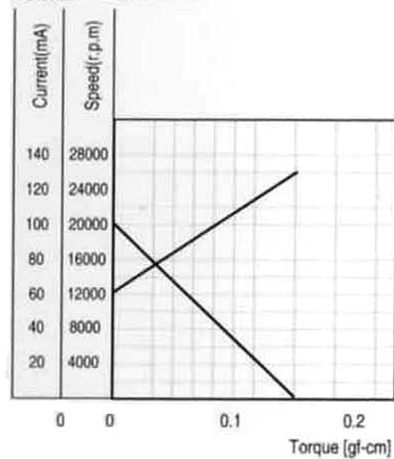
特性图 Characteristics
