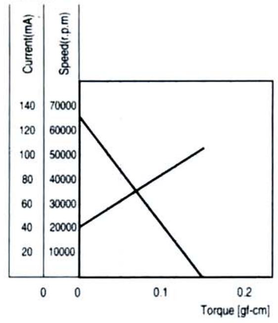
特性图 Characteristics
