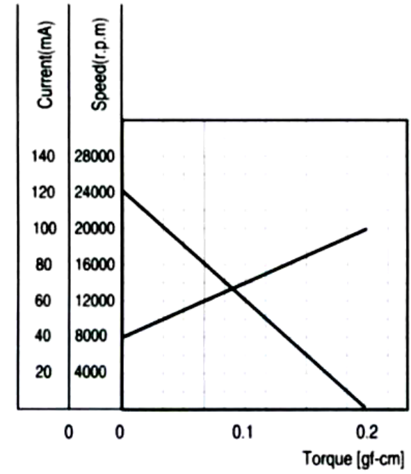
特性图 Characteristics
