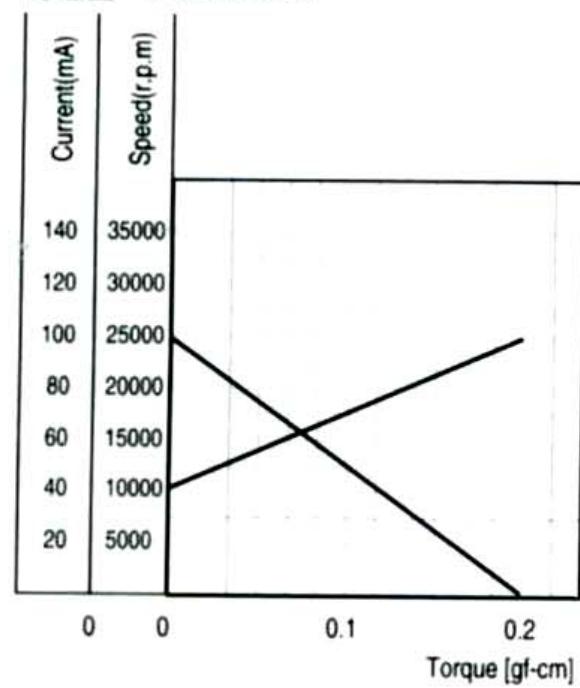
特性图 Characteristics
