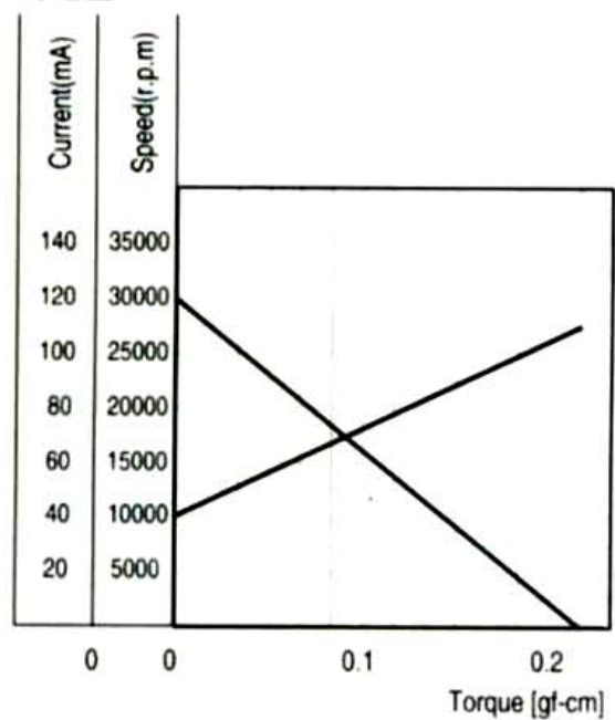
特性图 Characteristics
