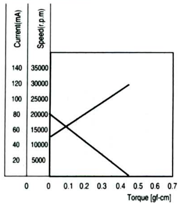
特性图 Characteristics
