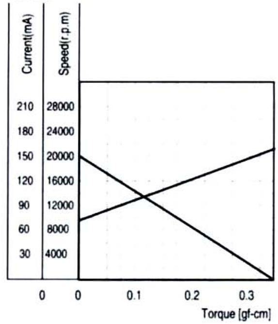
特性图 Characteristics
