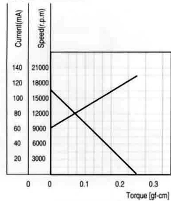
特性图 Characteristics
