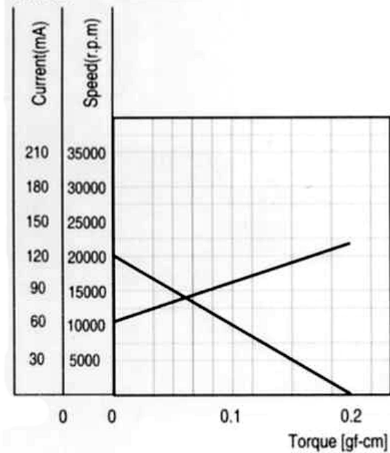
特性图 Characteristics
