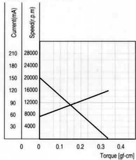
特性图 Characteristics
